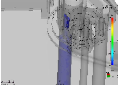
通过Moldflow分析生成位移量发生动画图
